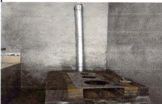
Foto 11 se construye la estufa rural en la cocina escolar
